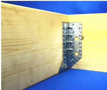
Typische Einbausituation
